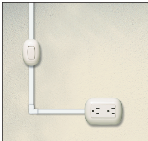
INSTALACIÓN CON MINICANALETAS Utilizando los adaptadores especiales de la línea OVAL®
